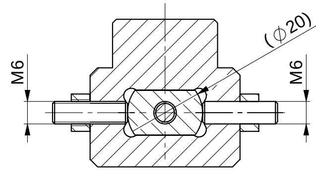
SEZIONE A-A
