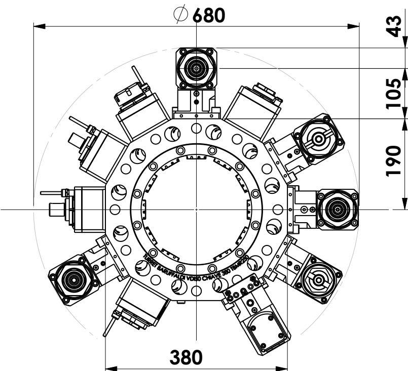
Gegenspindel COUNTERSPINDLE
