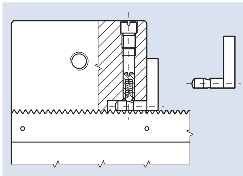
Satz Paralleleisen "Clak-System" bestehend aus 4 Paar Leisten
