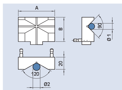
Prismenbacke mit "Clak-System"
