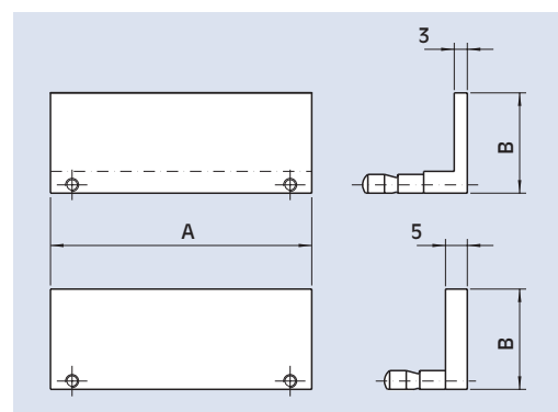
Satz Paralleleisen "Clak-System" bestehend aus 4 Paar Leisten
