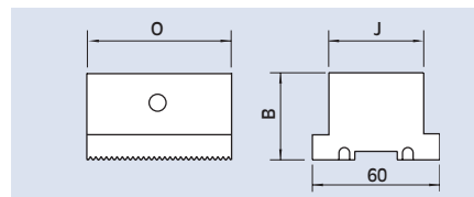
Fixbacken-Set mit Nutenstein Backenbreite J38
