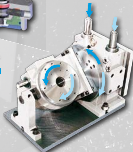
Touchdex-Rundtische für bis zu 5-Seiten-Bearbeitung in einer Aufspannung
